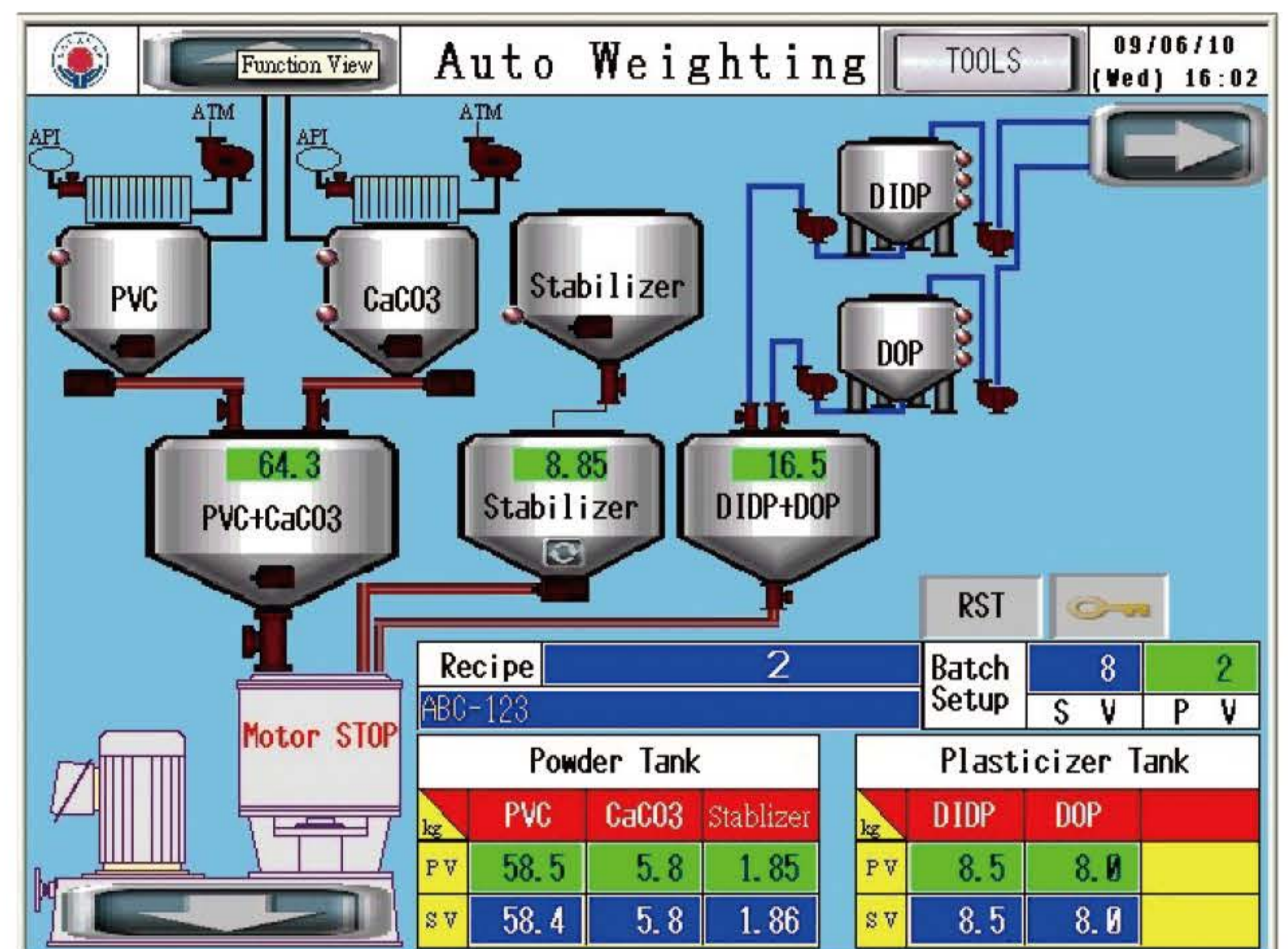
自動計量觸控式人機界面 Auto Weighting Control Panel
